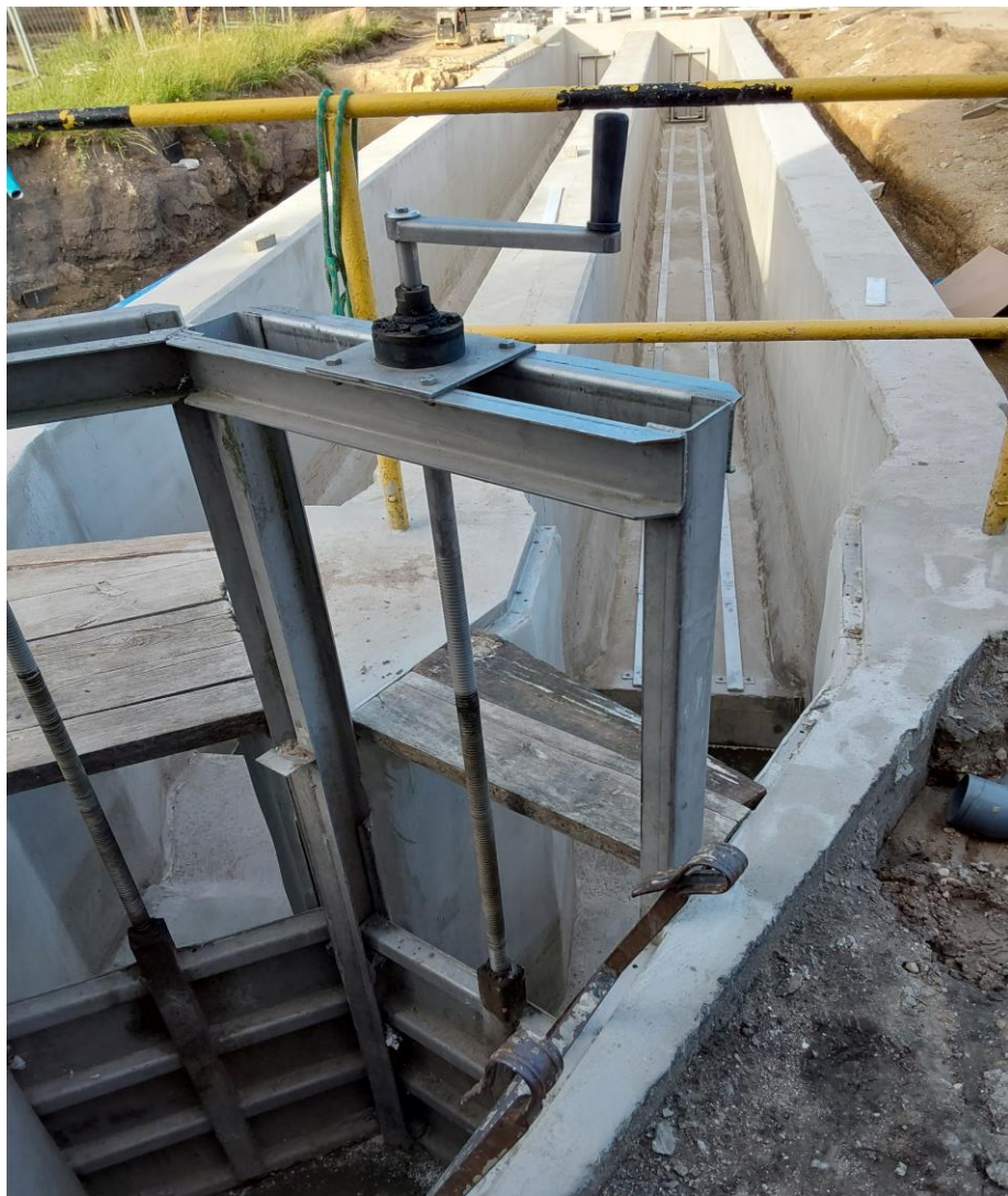
Przygotowanie piaskowników do montażu zgarniaczy, widok na nową elewację budynku krat na przepompowni
